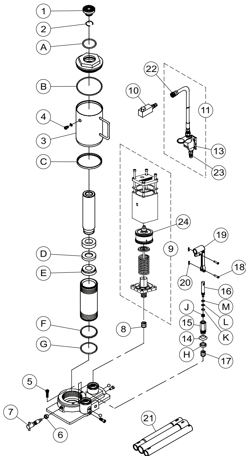
Figura 5: Ilustración de las piezas de repuesto para el modelo 18302C
