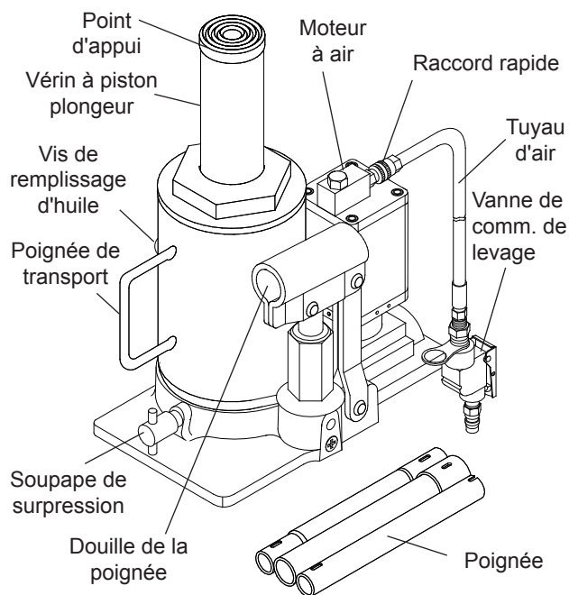
Figure 2 : Pièces du modèle 18302C
