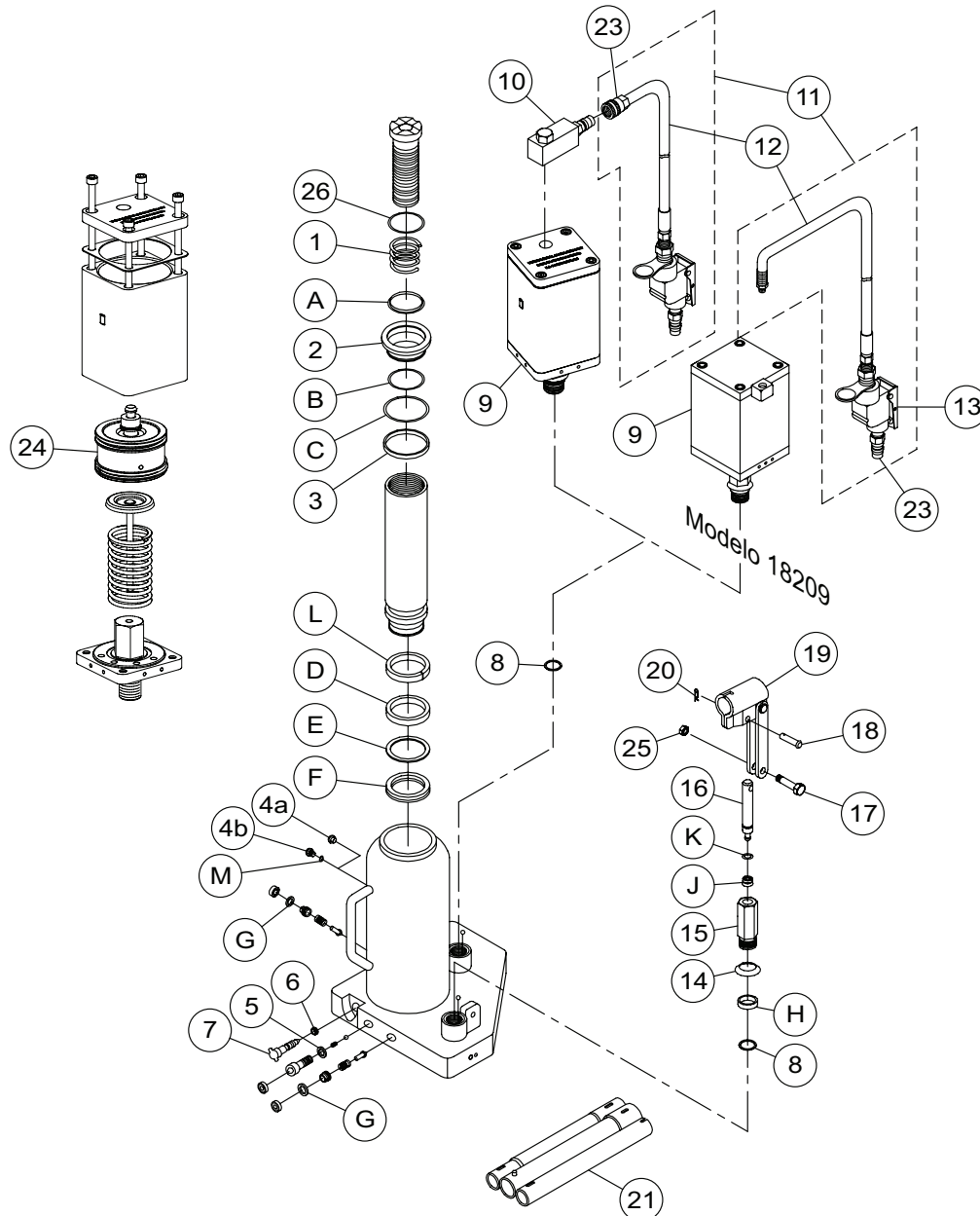
Figura 3: Ilustración de las piezas de repuesto para los modelos 18122C, 18202C y 18209
