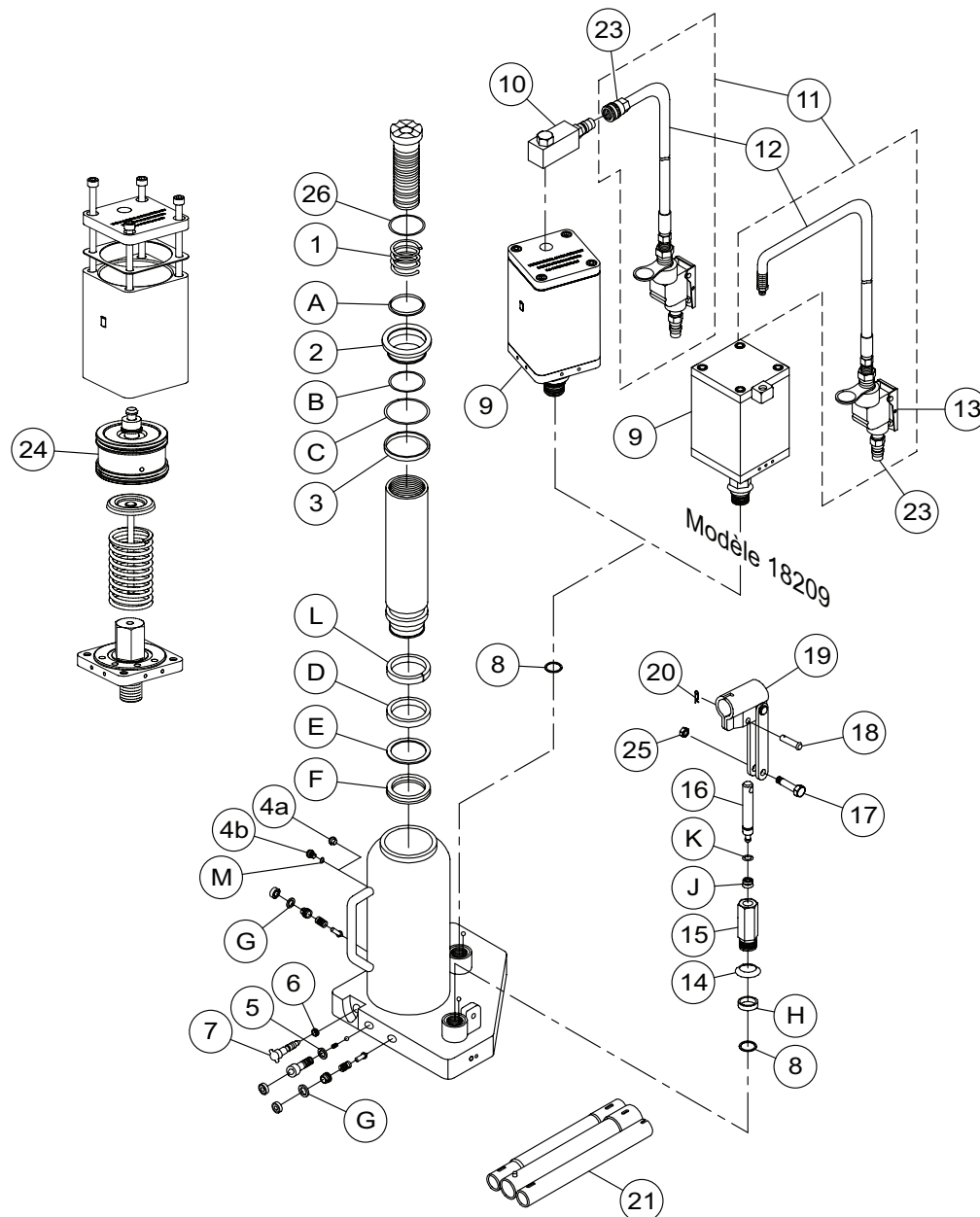
Figure 3 : Illustration des pièces de rechange des modèles 18122C, 18202C et 18209
