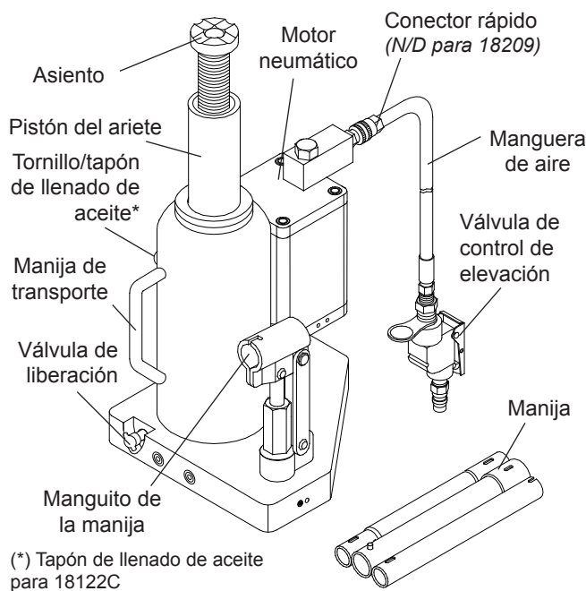
Figura 1: Nomenclatura de 18122C, 18202C, 18204C y 18209
