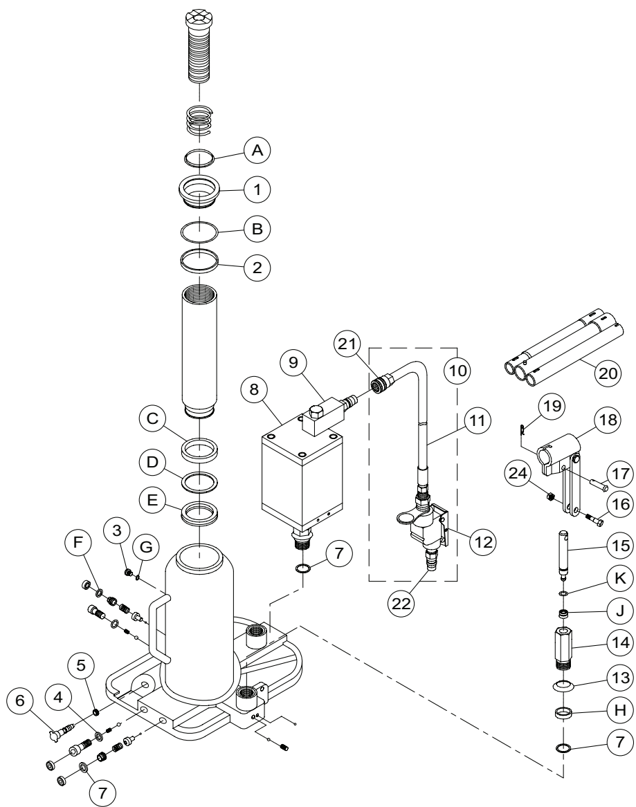
Figure 4 : Illustration des pièces de rechange du modèle 18204C
