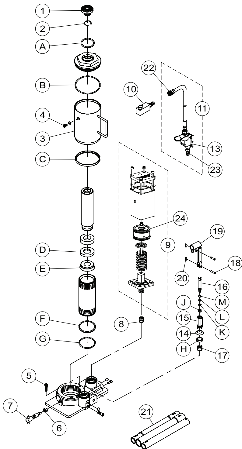
Figure 5 : Illustration des pièces de rechange du modèle 18302C
