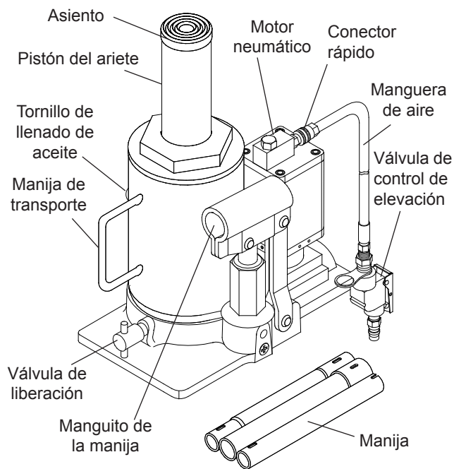
Figura 2: Nomenclatura de 18302C
