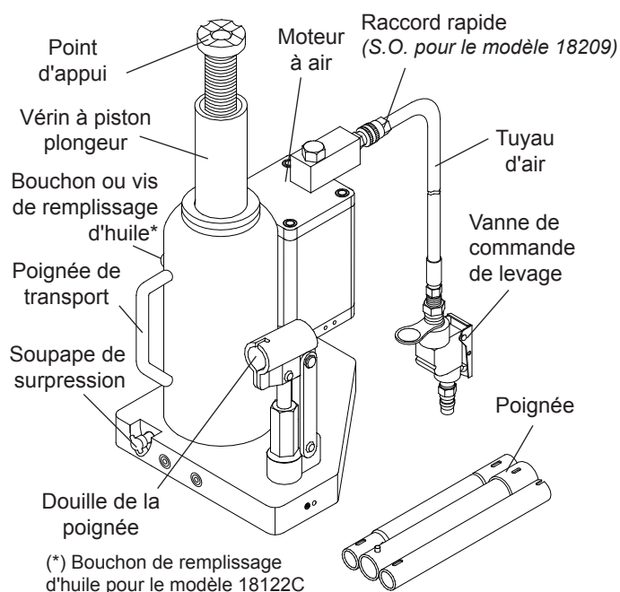
Figure 1 : Pièces des modèles 18122C, 18202C, 18204C et 18209
