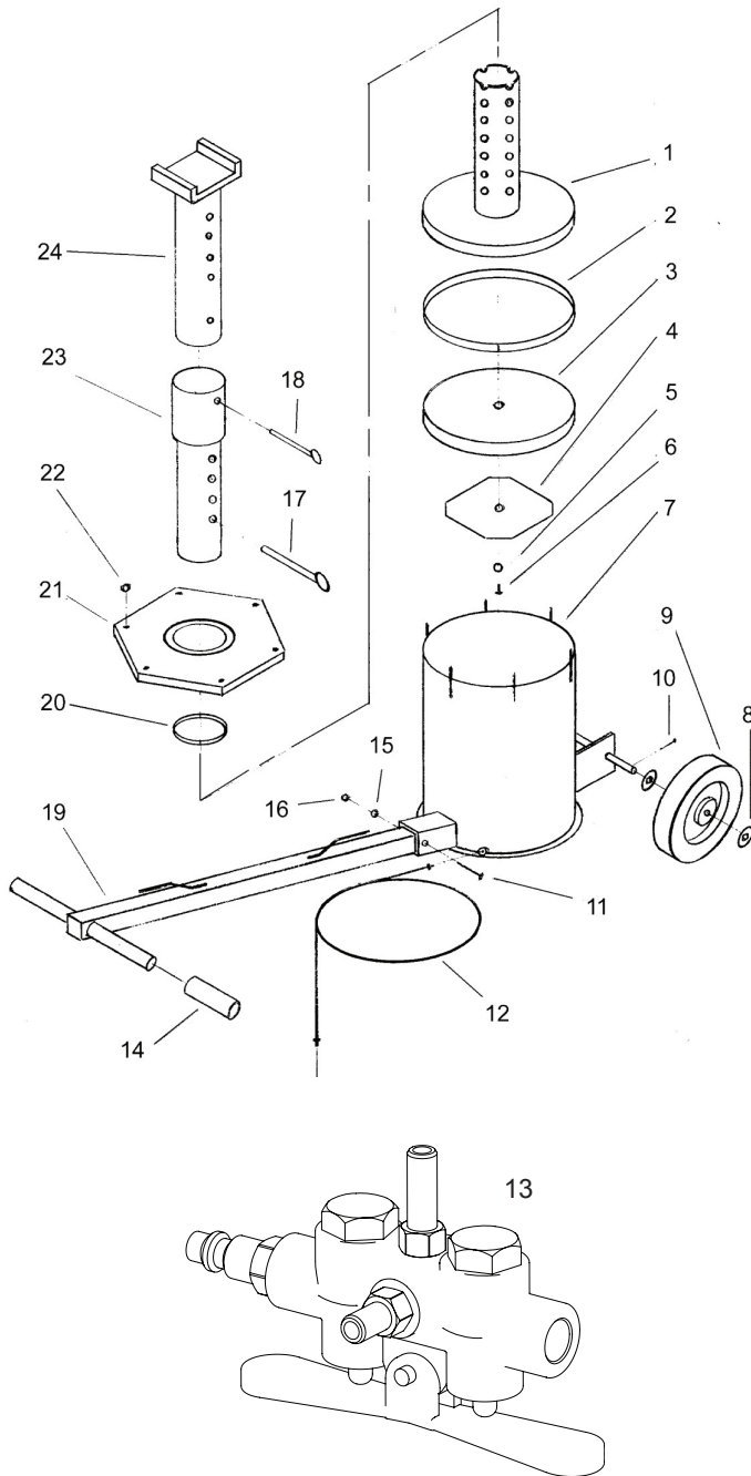
Figura 4: Ilustración de piezas para el modelo 34100
