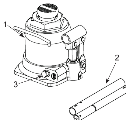
Figure 4 : Illustration pour les modèles BH2125B et BH2205B
