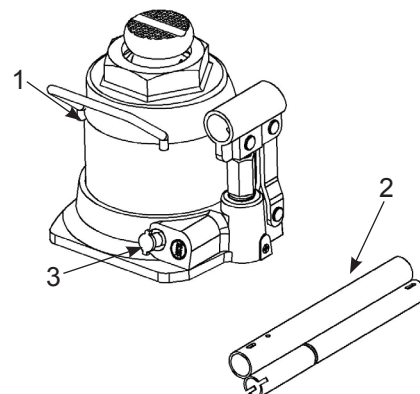
Figura 4: Ilustración para los modelos BH2125B y BH2205B
