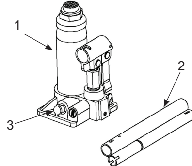
Figura 2: Ilustración para los modelos BH2020B, BH2040B y BH2060B
