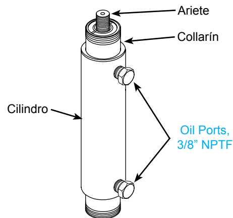
Figura 1: Componentes habituales del cilindro
