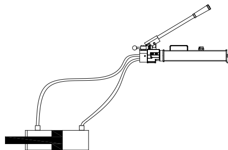
Figure 2 : Purger l'air du système
