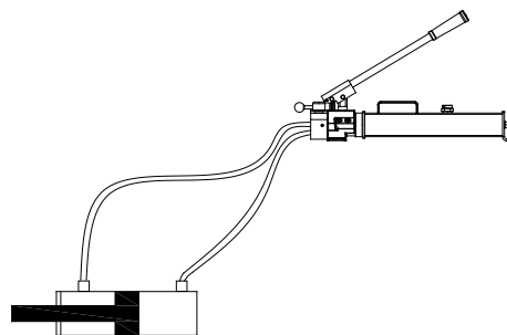
Figura 2: Ilustración de la purga de aire del sistema
